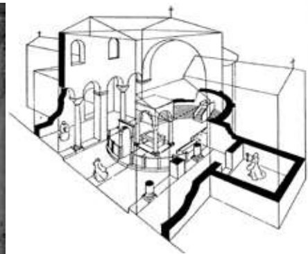
Ил. 6. Сирмиум, базилика Св. Димитрия. План, вид восточной части, аксонометрическая реконструкция (Jeremiћ 2003: 47, 50)
