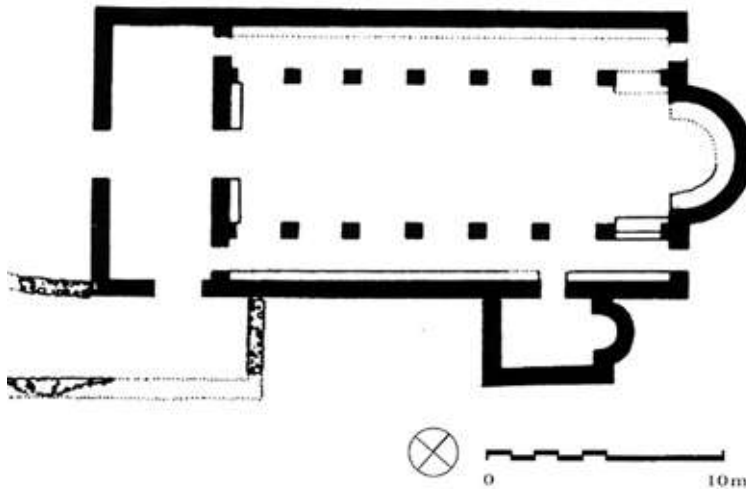
Ил. 11. Крепость Арса. План базилики (Ćurčić 2010: 226)
