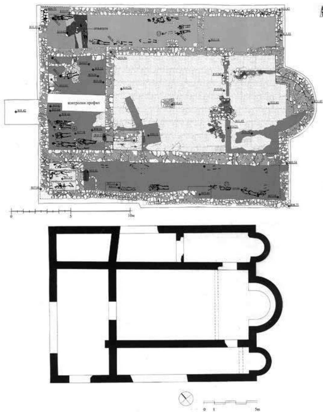
Ил. 14. Градина на Елице. Планы базилик D (сверху) и А (снизу) (Милинковић 2010: 297; Ćurčić 2010: 225)
