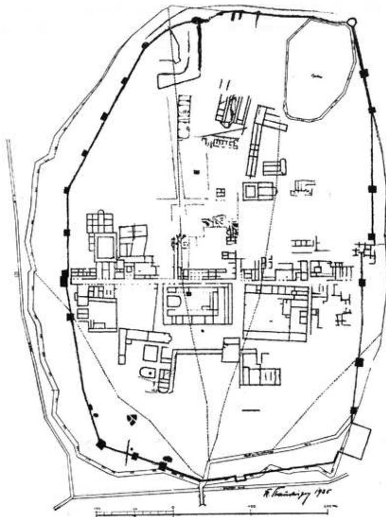
Ил. 4. Крепость Бассиана. План (Васић 2013: 82 по Грбић 1936: сл. 2)
