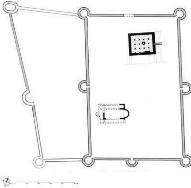
Ил. 9. Крепость Балайнац. План (Ćurčić 2010: 181)
